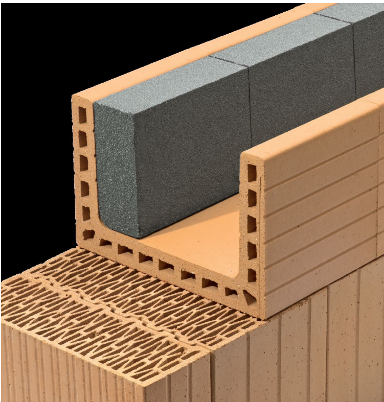
WGU-Schalen als Ringanker...
