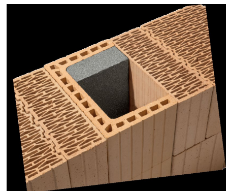
... als Schalung für integrierte Stürze
